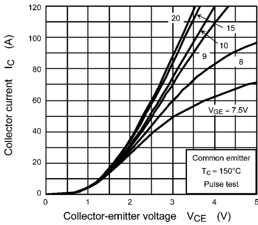
Fig. 8.3 I_C - V_{CE}
