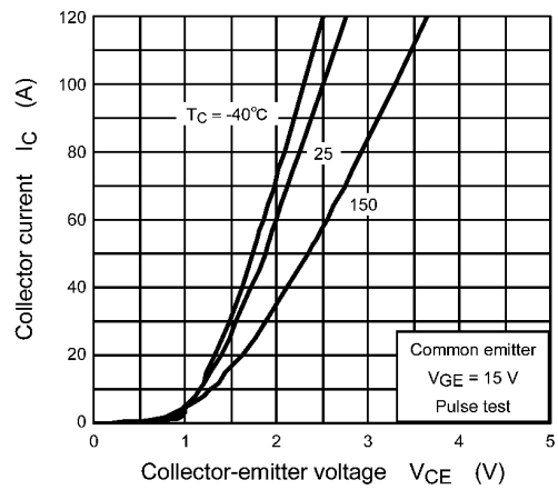
Fig. 8.4 I_C - V_{CE}
