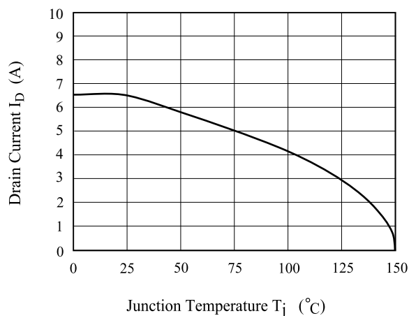
Fig10. I_D - T_j
