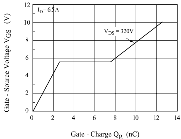
Fig8. Q_g - V_{GS}
