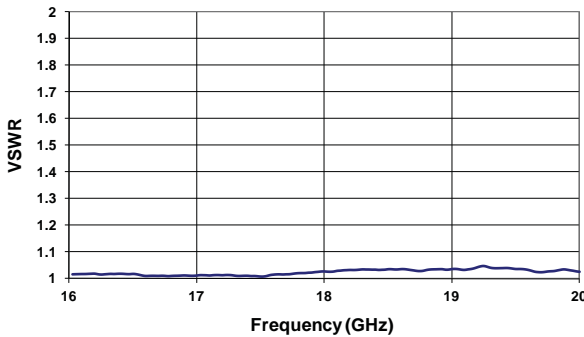
VSWR ( 16-20 GHz )
