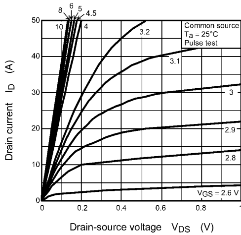
Fig. 8.1 I_D - V_{DS}
