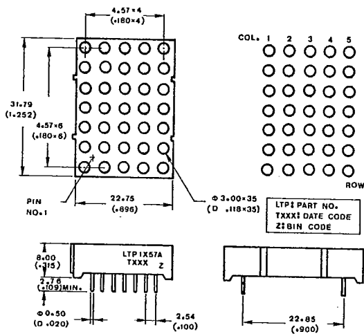
B. LTP-1457A/1557A
