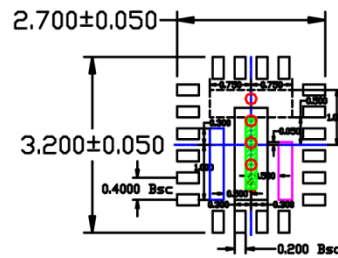
BOTTOM VIEW NOTE : 1,2,3
