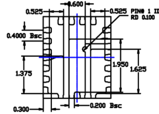
BOTTOM VIEW NOTE : 1,2,3
