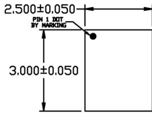
TOP VIEW NOTE : 1,2,3
