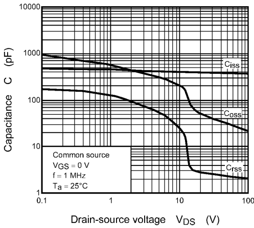
Fig. 8.9 C - V_{DS}
