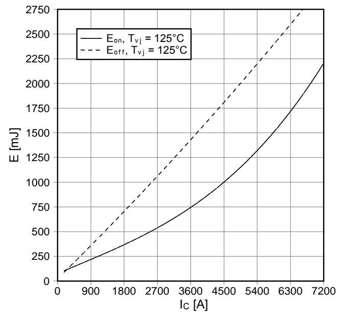
Schaltverluste IGBT-Wechselr. (typisch) switching losses IGBT-inverter (typical) E_{on} = f(I_c) , E_{off} = f(I_c) V_{GE} = \pm 15\text{ V} , R_{Gon} = 0,4\ \Omega , R_{Goff} = 0,5\ \Omega , V_{CE} = 900\text{ V}
