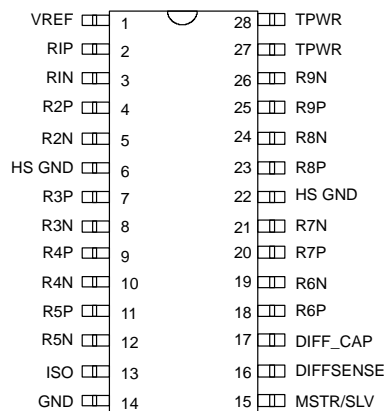
DS2119MB 28-PIN TSSOP
