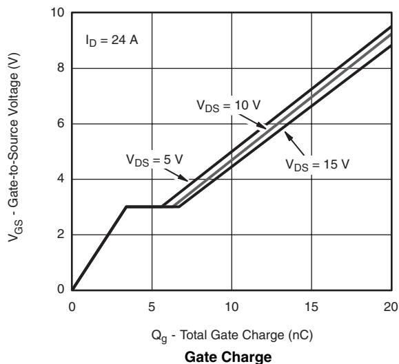
I_D = 24\text{ A} V_{DS} = 10\text{ V} V_{DS} = 5\text{ V} V_{DS} = 15\text{ V} Gate Charge
