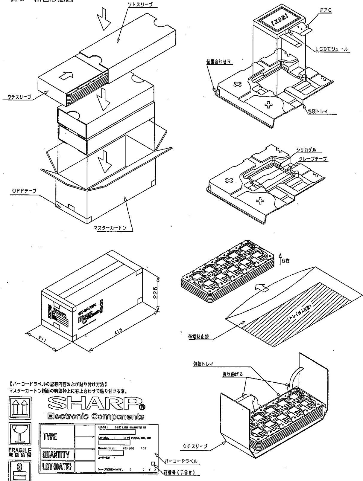
図3 梱包形態図
