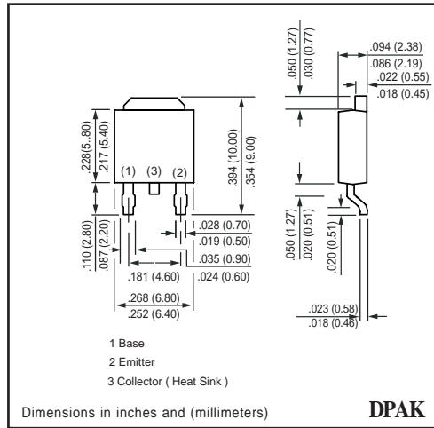
DPAK
