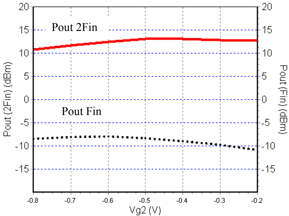
Pout (2Fin) & Pout (Fin) vs Vg2 for Fin = 12 GHz, Pin=14dBm & Vg1= -0,9V
