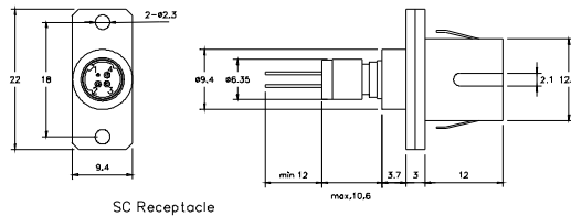
SC Receptacle
