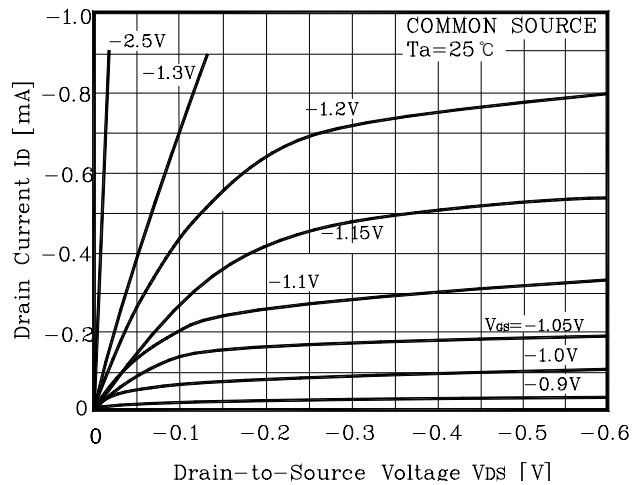
Fig2 I D - V DS
