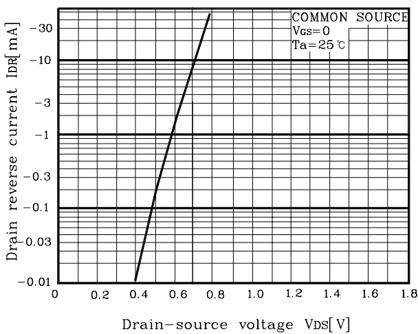
Fig3 I DR - V DS
