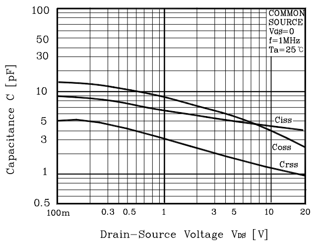
Fig.6 C - V_{DS}
