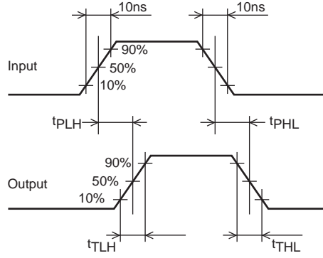
スイッチングタイム波形図
