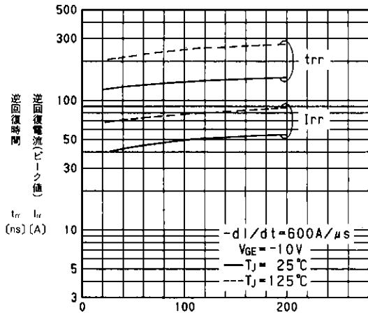
ダイオード順電流 I c (A) Trr, Irr-Ic特性 Trr, Irr-Ic
