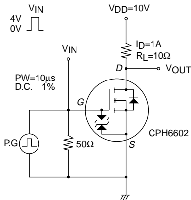
スイッチングタイム測定回路図
