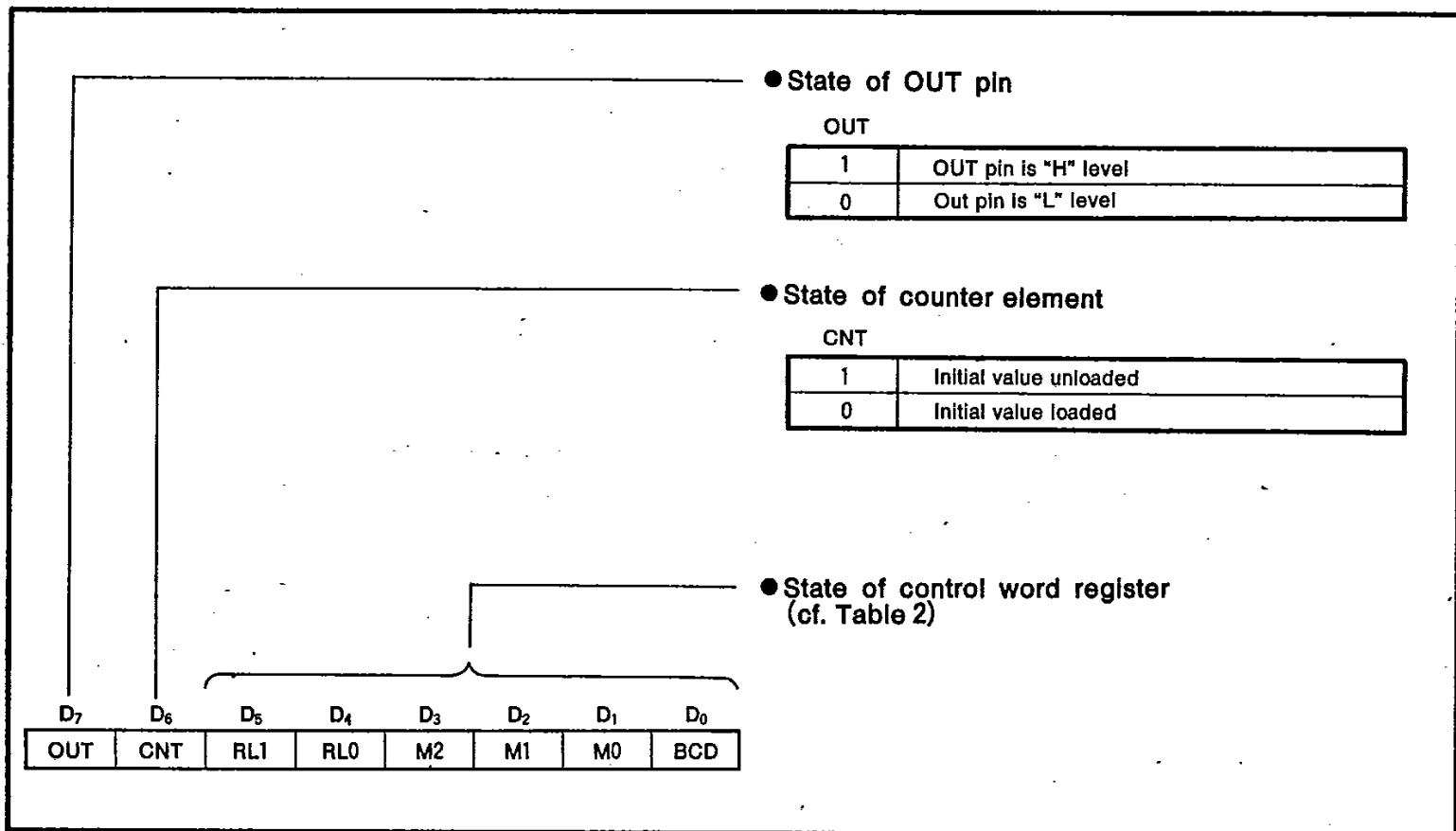
Fig. 9 Status Byte
